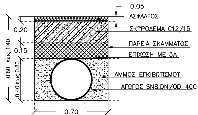
ΤΥΠΙΚΗ ΔΙΑΤΟΜΗ 3
