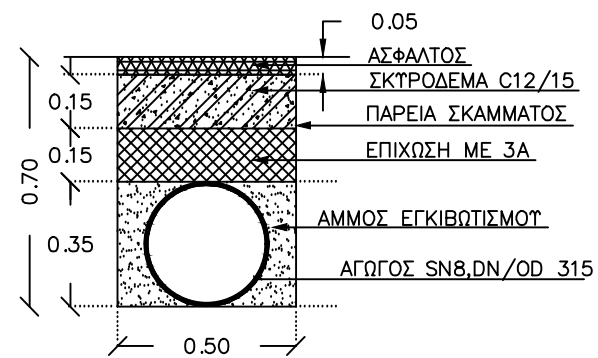
ΤΥΠΙΚΗ ΔΙΑΤΟΜΗ 2
