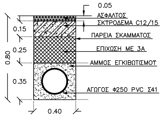
ΤΥΠΙΚΗ ΔΙΑΤΟΜΗ 1
